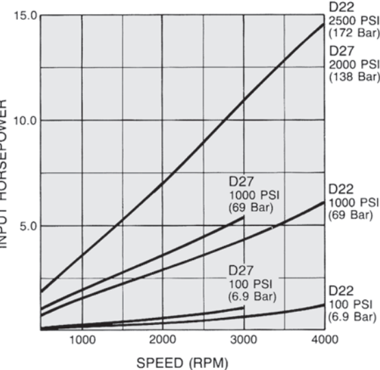
D22/D27 Horsepower/Speed
