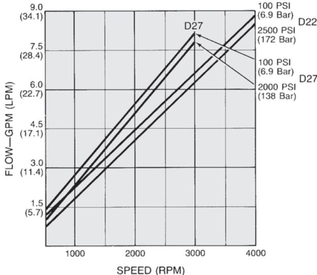
D22/D27 Flow/Speed
