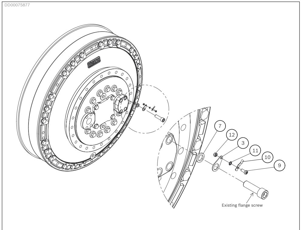
Fig. 9: Grounding point example, Hägglunds Viking 84
