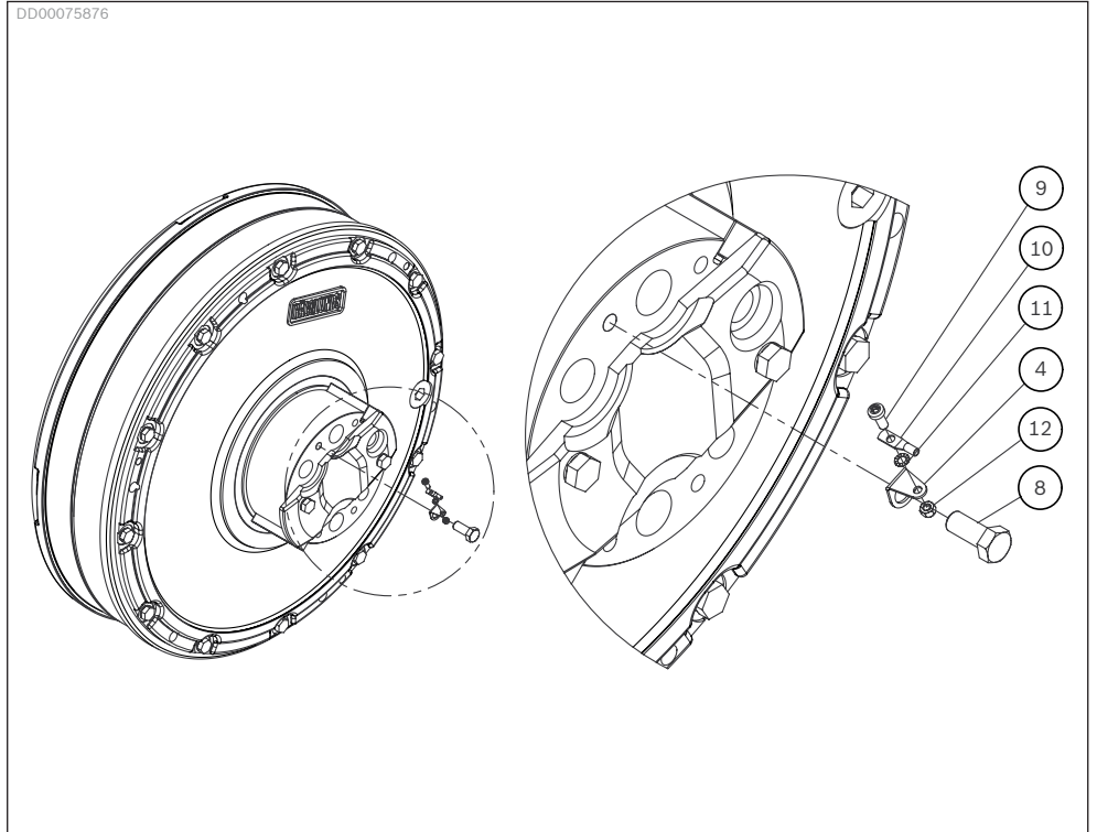
Fig. 8: Grounding point example, Hägglunds Viking 44/64
