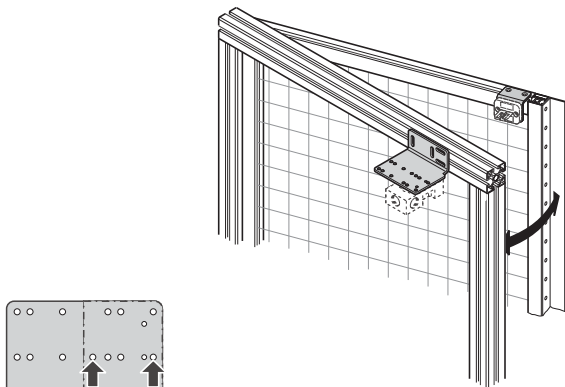
Schmersal AZ 15... Schmersal AZ 16...
