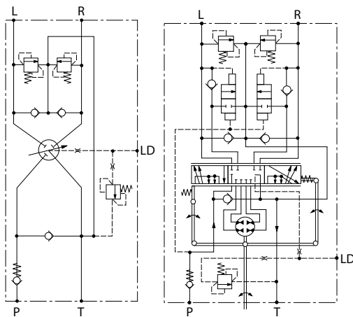
Figure 4: LAGU LD / NR schematic
