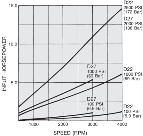
D22/D27 Horsepower/Speed
