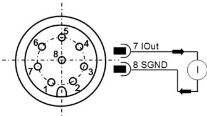
Fig. 3: Mesure des sorties analogiques 4...20 mA sans résistance de charge
