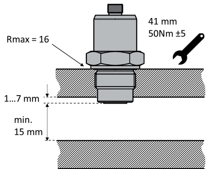
Fig. 1: Montage du capteur et rayon de détection
