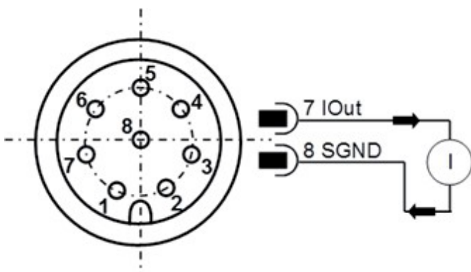
Ilustración 3: Medición de la salida analógica 4 ... 20 mA sin resistencia de carga
