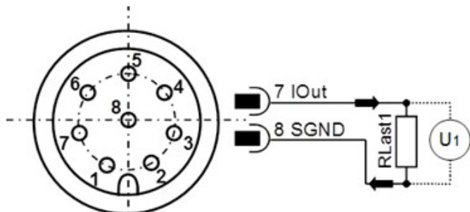
图4: 连接负载电阻以测量4...20 mA模拟输出
